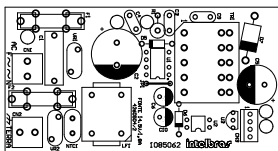
Fonte AC
